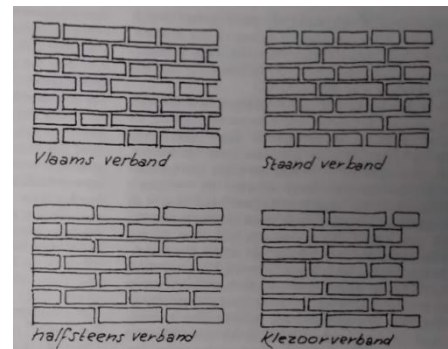
Voorbeelden van metselverbanden
